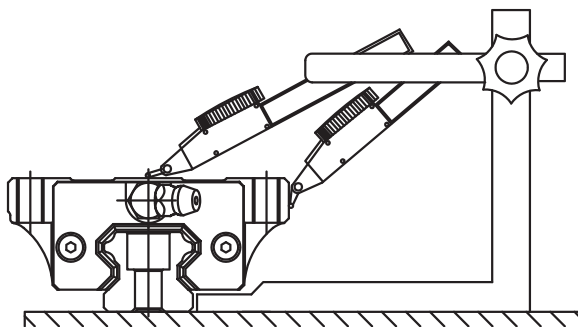
(圖 1) 行走平行度的量測
