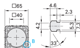
A-A View
