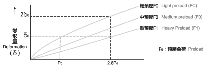
(圖 2) 剛性 (fig.2) Stiffness
