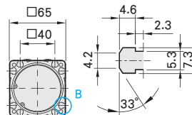
A-A View
