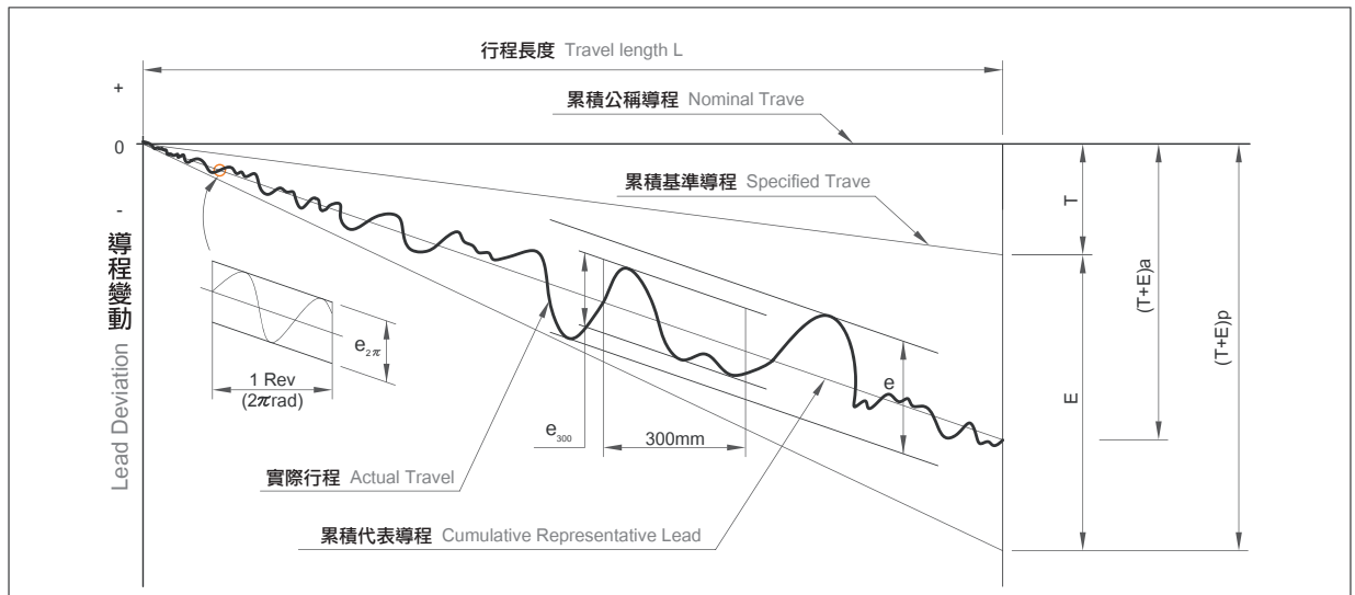
圖 1 導程量測曲線 Fig.1 Technical Terms Concerning the Lead
